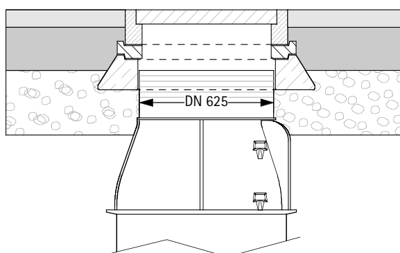
Betonowy pierścień odciążający
